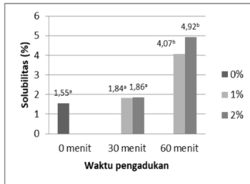
Gambar 9 Pengaruh penambahan STPP (0%, 1%, 2%) dan waktu pengadukan (0 menit, 30 menit, 60 menit) terhadap solubilitas
