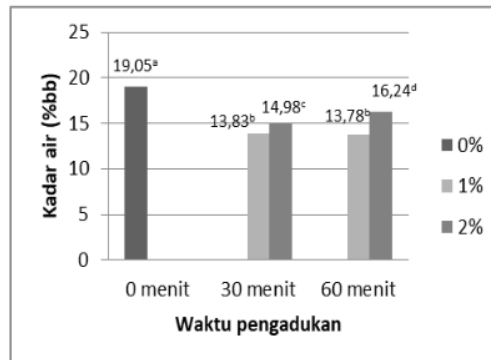
Gambar 4 Pengaruh penambahan STPP (0%, 1%, 2%) dan waktu pengadukan (0 menit, 30 menit, 60 menit) terhadap kadar air.
