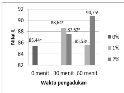
Gambar 1 Pengaruh penambahan konsentrasi STPP (0%, 1%, 2%) dan waktu pengadukan (0 menit, 30 menit, 60 menit) terhadap nilai warna (L).
