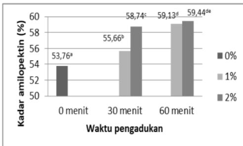
Gambar 7 Pengaruh penambahan STPP (0%, 1%, 2%) dan waktu pengadukan (0 menit, 30 menit, 60 menit) terhadap kadar amilopektin
