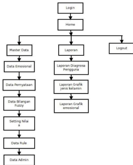
Gambar 4. Peta situs level pengguna.
